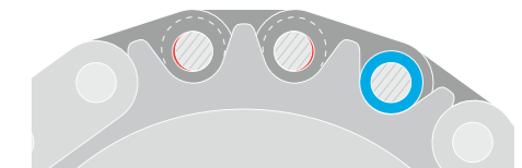
Durch den Verschleiß an den Bolzen und in den Hülsen kann sich die Steuerkette längen.
